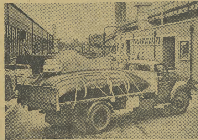
Niedawno zamieściliśmy zdjęcie nylonowych pojemników do transportu płynów drogą wodną, dziś reproduujemy zdjęcie pomysłowego zbiornika z plastyku, który eliminuje auta — czy też wagonycysterny, można go bowiem stosować w połączeniu z dowolnym środkiem lokomocji. Jest przy tym łatwy do przechowywania, gdyż daje się zgrabnie zwijać w naciągany namiot. Nazwano go „Portolite” i ma pojemność 800 galonów. Projekt angielskich inżynierów. (db)
