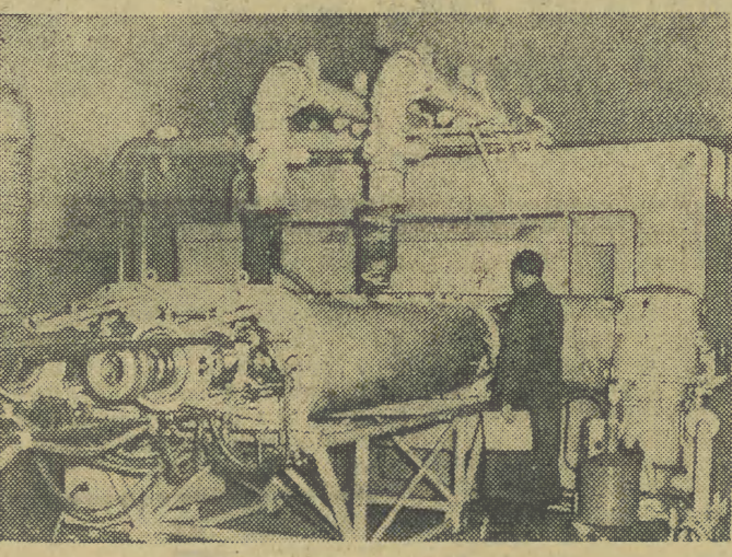
Cyklotron. Widać elektromagnes, komorę akceleracyjną i linie rezonansowe z pompami próżniowymi. Proces przyspieszania cząstek wymaga warunków wysokiej próżni.
