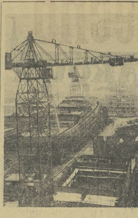
Stocznia szczeecińska rozpoczęła produkcję w 1931 roku. Od tego czasu wodowano już 32 jednostki, a trzydziesta trzecia zostanie spużzona na wodę w najbliższym czasie. Dotychczas stocznia produkowała rudo- wogłowce typu B-32 o nośności 3200 ton. Obecnie przystąpiono do budowy jednostki motorowej o nośności 6000 ton. Na zdjęciu: Rudowogłowiec typu B-32 na pochylni stoczni.
