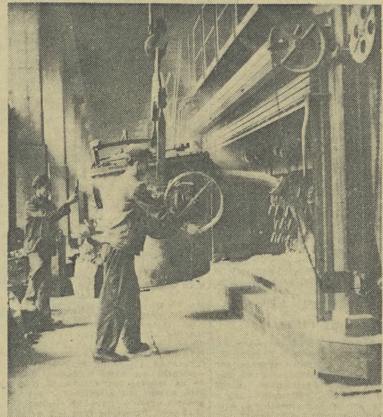
Na zdjęciu: Stanisław Bałazy i Julian Burda wyciągają płynne aluminium z wanny przy pomocy kadzi próżniowej. CAF fot. Link
