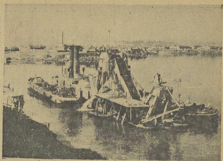
UŻ na wiosnę przyszłego roku zostanie oddany do użytku Kanał Wołga - Don—wielka budowla komunizmu ZSRR. Na zdjęciu fragment prac przy budowie kanału.
