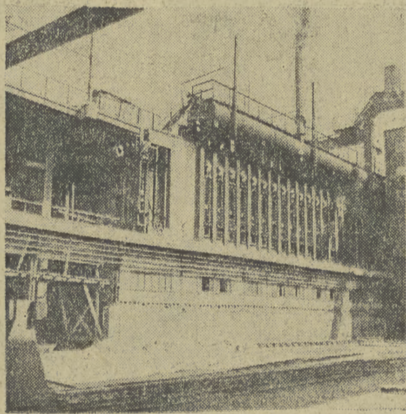
Z lewej: budowa nowej koksowni huty „Kościusko” w Chorzowie. Z prawej: fragment nowo wybudowanej baterii koksowni w Gliwicach.
