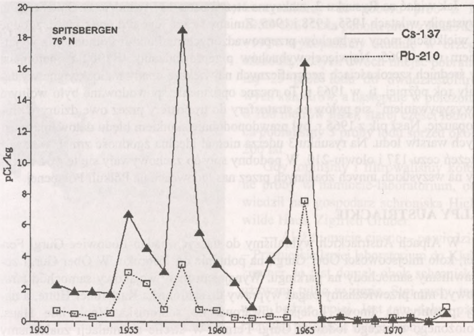
Rysunek 3. Stężenia cezu-137 i ołowiu-210 w Lodowcu Köbera na Spitsbergenie.
