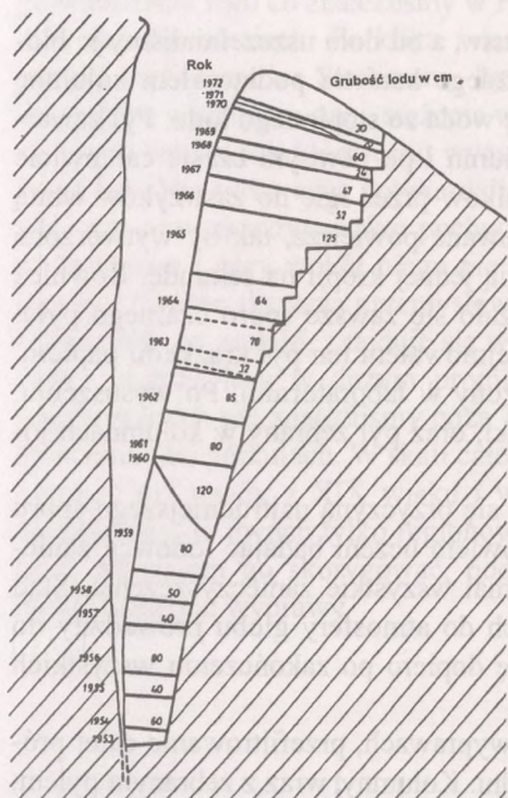
Rysunek 2. Przekrój wykopu w szczelinie lodowca Storbreen, Norwegia.
