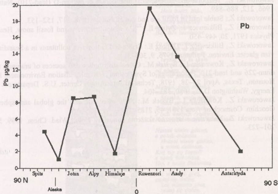
Rysunek 5. Równoleżnikowy rozkład średnich stężeń ołowiu trwałego we współczesnym lodzie lodowcowym.
