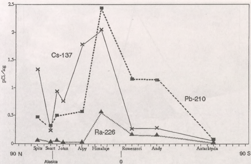
Rysunek 4. Równoleżnikowy rozkład średnich stężeń ołowiu-210, cezu-137 i radu-226 we współczesnym lodzie lodowcowym, pomiędzy szerokością geograficzną N 76,02° i S 62,05°.
