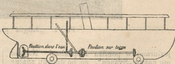
Fig. 3. Przecięcie schematyczne „Łabędzia”. Linia cieniowana przedstawia mechanizm transmisji na wodzie, linia jasna na lądzie.
