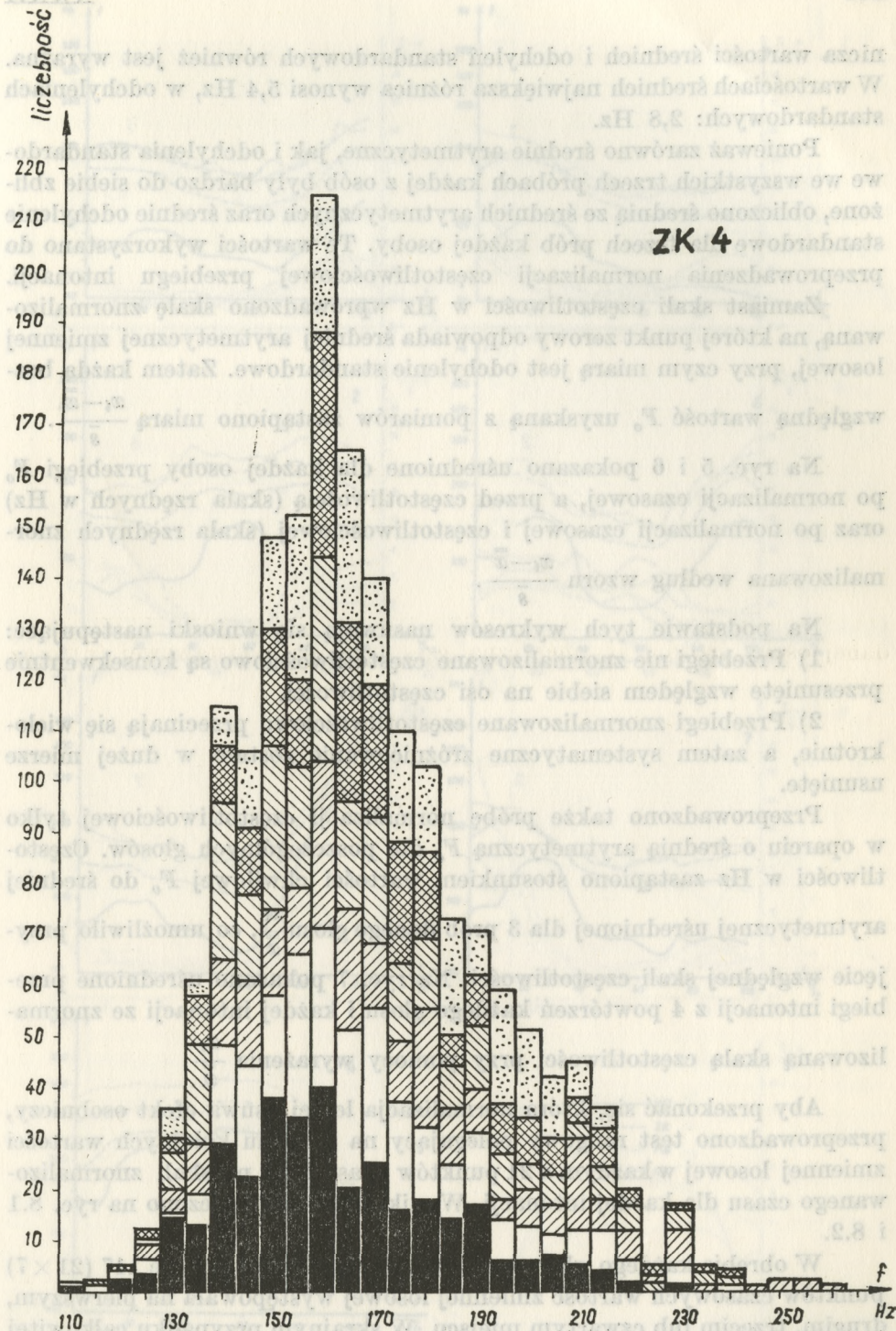
Ryc. 4. Histogram wartości chwilowych F_0 jednej wersji jednogminutowego tekstu wymówionego przez jedną osobę sporządzony co 10 s.
