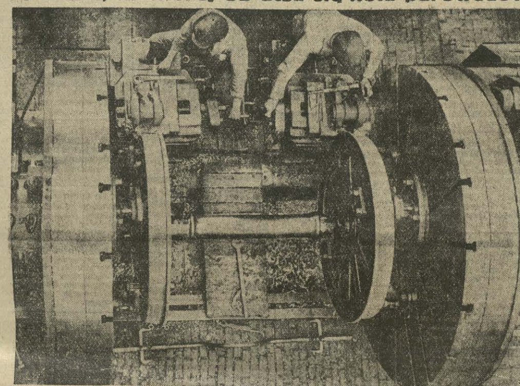
Jest to olbrzymia, jak widać, obrabiarka, służy ona do obtaczania kół parowozowych o średnicy 1.50 m. Czynna jest w jednej z angielskich fabryk parowozów.
