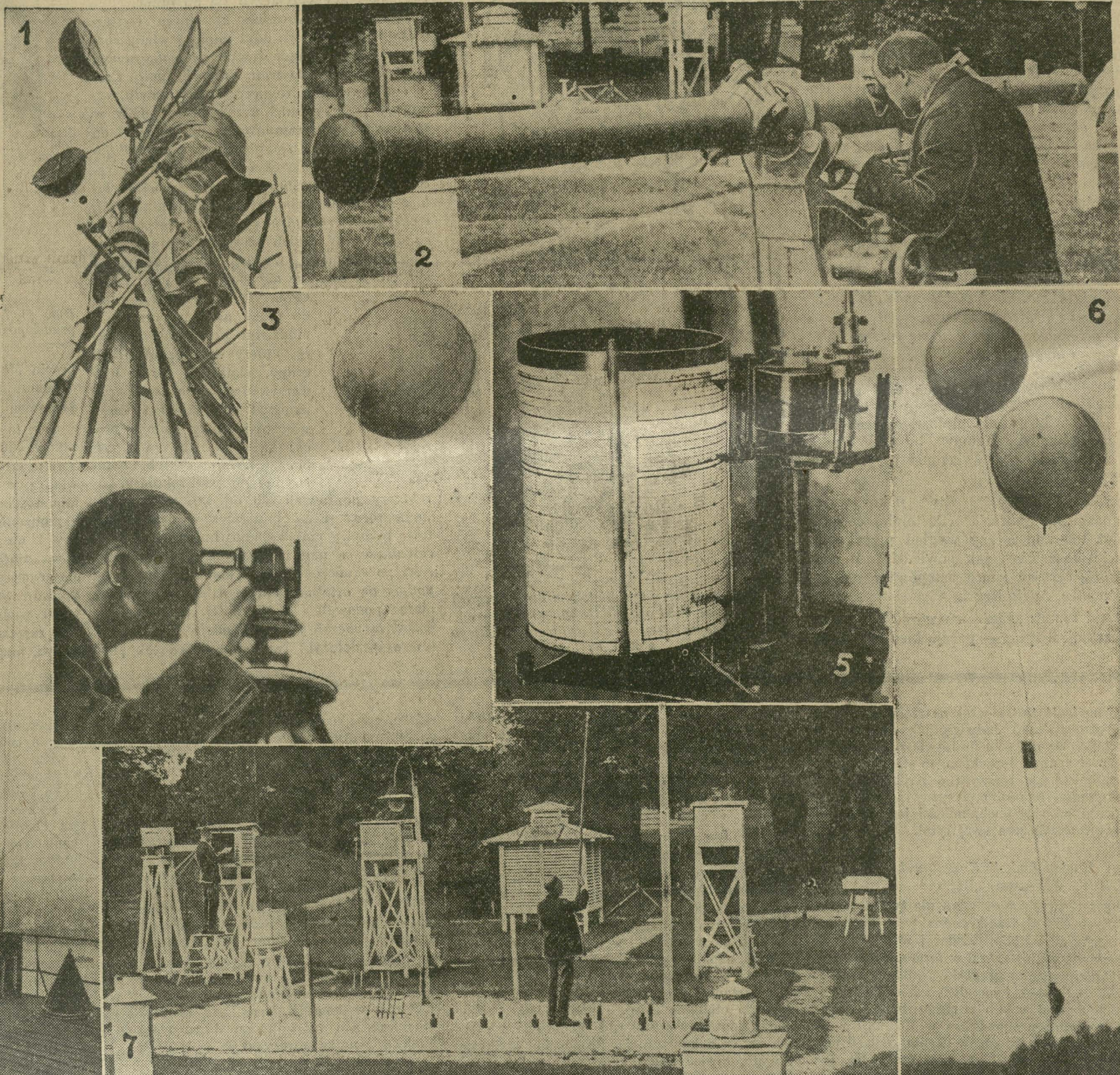
Rys. 1) Zewnętrzna część anemografu, umieszczonego na szczycie masztu okrętowego. Widać potężne łyżki obrotowe, rejestrujące szybkość wiatru i strzałę, wskazującą kierunek wiatru. — Rys. 2) Stereotelegraf, służący do mierzenia odległości (w tym wypadku chmur) mający odstęp soczewek 4 m., co pozwala na pomiar odległości 25 km. — Rys. 3) Dla badania prądów (wiatrów) w górnych częściach atmosfery wypuszcza się baloniki gumowe, których lot oznacza się co minutę przy pomocy teodolitu. — Rys. 4) Maszt okrętowy w porcie w Hamburgu (z tyłu widok na miasto), na którym wywiesza się sygnały przepowiadające pogodę. — Rys. 5) Wewnętrzna część anemografu rejestrująca ruchami szybkość i kierunek wiatru. — Rys. 6) Dla badania górnych warstw atmosfery wysyła się w górę przy pomocy balonów meteorograf samonotujący zmiany temperatury ciśnienia i wilgotności w górnych częściach atmosfery. — Rys. 7) Widok ogólny na meteorologiczną stację w Potsdamie. Na planie drugim umieszczone są klatki termometryczne z przyrządami samopiszącymi. Z tyłu ewaporometr (kształtu miednicy). Na pierwszym planie opadomierz. W pośrodku widać geotermometry, z których jeden trzyma w ręce obserwator.
