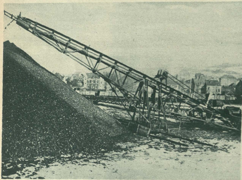
Z wielkich kopalń węgla. Zdjęcie nasze przedstawia nowy lewar, używany w sławnych niemieckich kopalniach w Essen, a umożliwiający daleko szybszą eksploatację. Niemcy tym węglem głównie płacą swoje długie wojenne.
