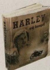
Wojciech Echilczuk, Tomasz Szczerbicki , „Harley mój kumpel”, Warszawa 2008, s. 432, 145 zł
