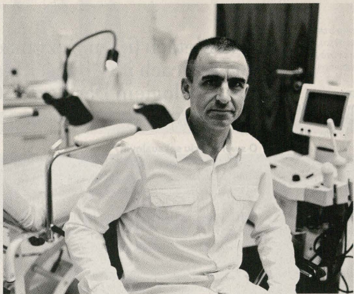
Doktor nauk medycznych Dariusz Góral
