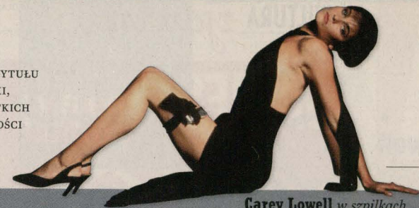
Carey Lowell w szpilkach
