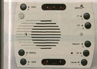
Jedne z modułów systemu IDRA. Niewiele większy od kontaktu łączy w sobie między innymi funkcje czujnika temperatury i światła, interkomu oraz transmitera przekazującego sygnały w podczerwieni. Takie elementy rozmieszczone w całym domu łączą się kablami, przez które przekazują sygnały między sobą oraz wprost do serca systemu – domowego komputera
