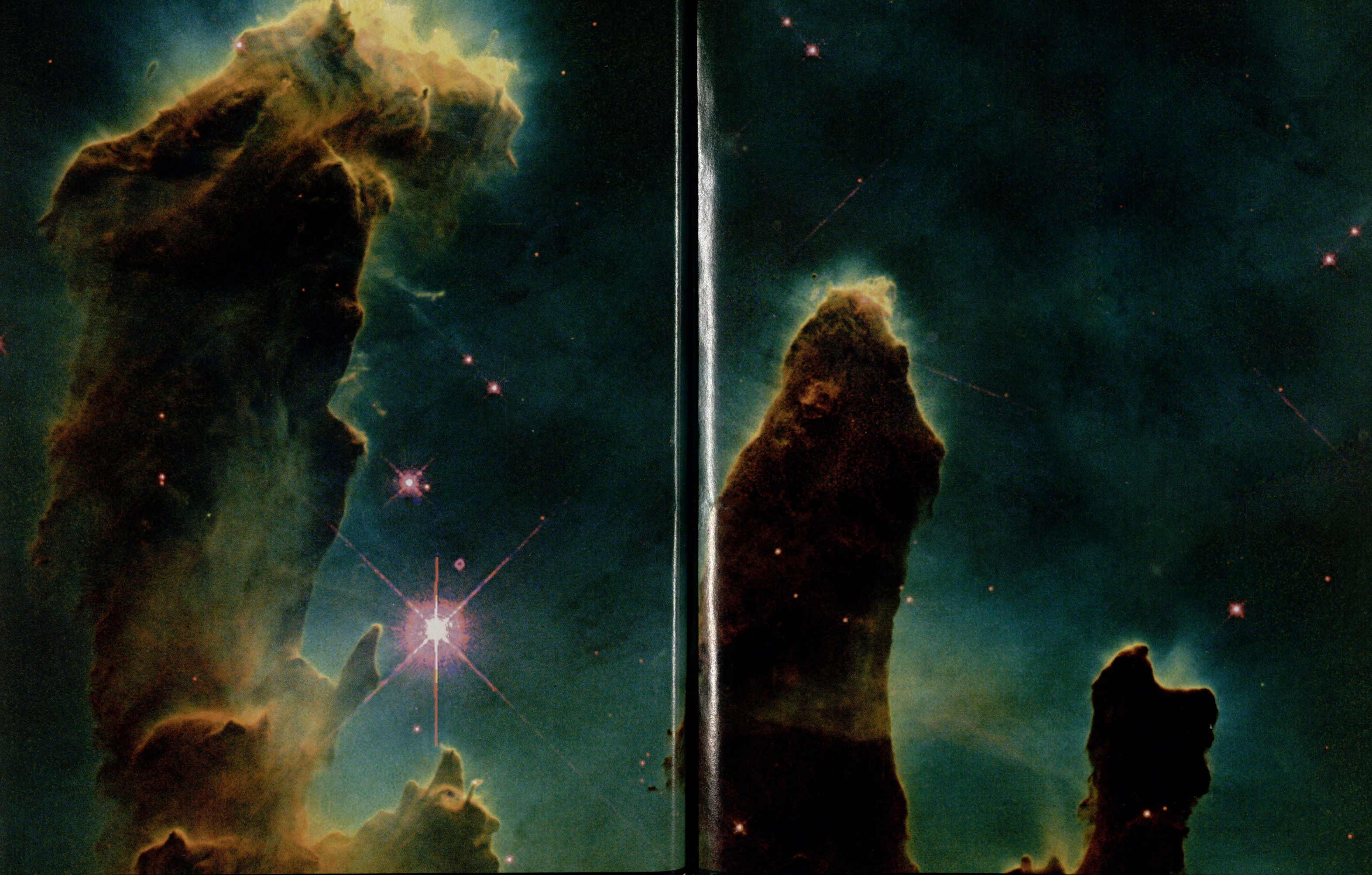
FILARY STWORZENIA – GIGANTYCZNE KOLUMNY GAZU I PYŁU LEŻĄCE W MGŁAWICY ORZEŁA. TO ZALEDWIE 6.5 TYSIACA LAT ŚWIETLNYCH OD ZIEMI
