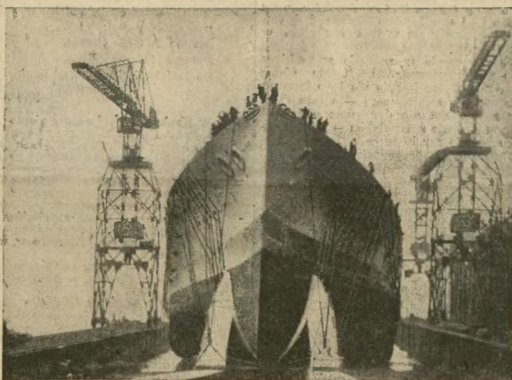
W Newcastle w obecności króla Jerzego VI, spuszczonej został na wodę nowy brytyjski okręt wojenny, który otrzymał nazwę „Jerzy VI”. Zdjęcie na lewo przedstawia króla Jerzego VI podczas ceremonii chrztu okrętu; na prawo: kadłub okrętu.
