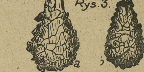
Rys. 3): a. domek otwornicy Diffugia ; b. domek sztucznie otrzymany.
