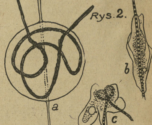
Rys. 2): a. „Polykanie“ nitki szelaka przez kroplę chloroformu, b, c, polykanie nitki wodorostu przez amoebę.
