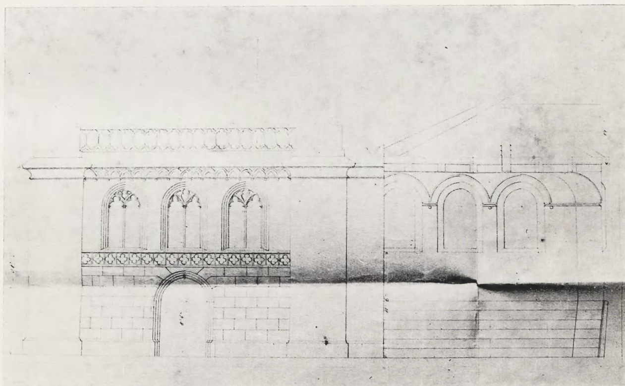
3. Projekt budowy rajtszuli z 1826 r., elewacja
