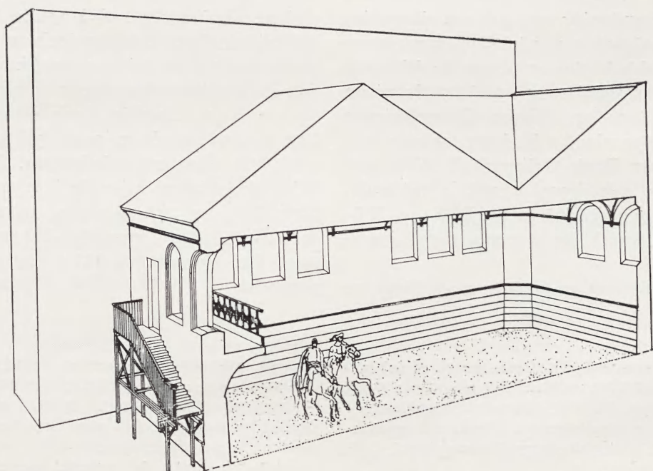
7. Rekonstrukcja rajtszuli według projektu z 1826 r., wewnątrz
