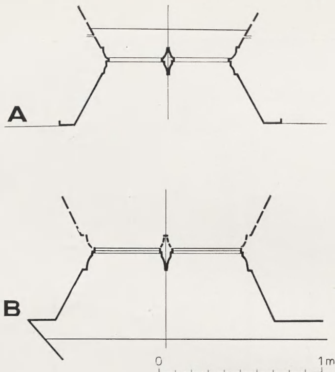
3. Przekroje poziome okien dwu gotyckich kaplic katedry na Wawelu: A — kaplica Św. Małgorzaty (okno odsłonięte w r. 1981), B — kaplica Św. Katarzyny (obecnie Zakrystia). Oprac. P. Stępień
