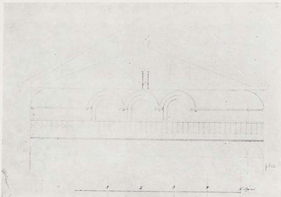
4. Projekt budowy rajtszuli z 1826 r., ściana z antresolą
