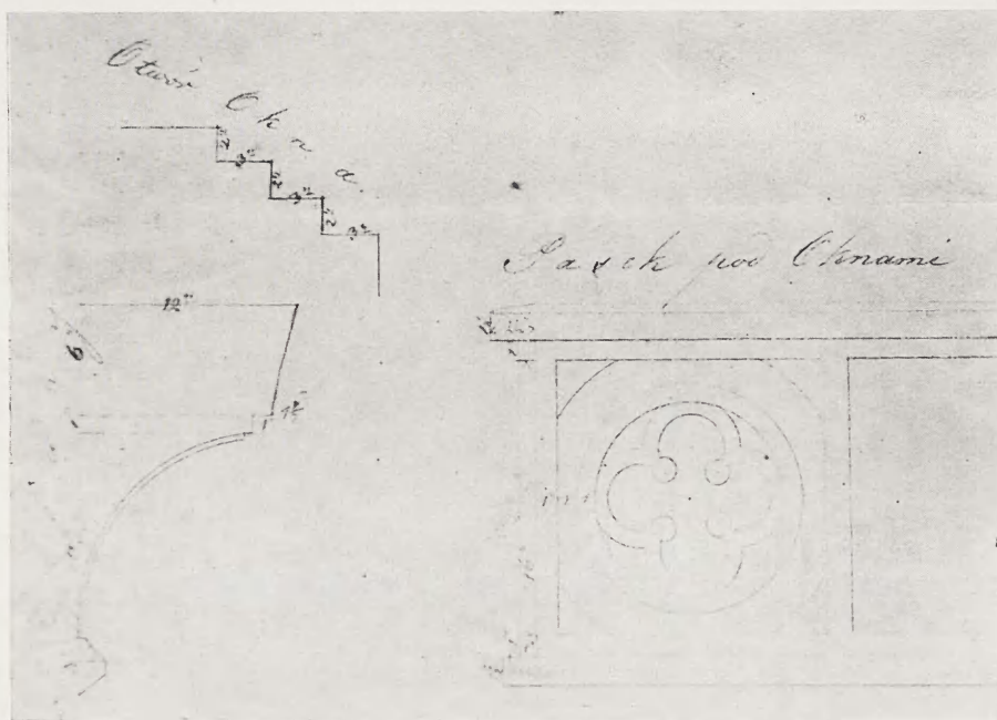
5. Projekt budowy rajtszuli z 1826 r., detale
