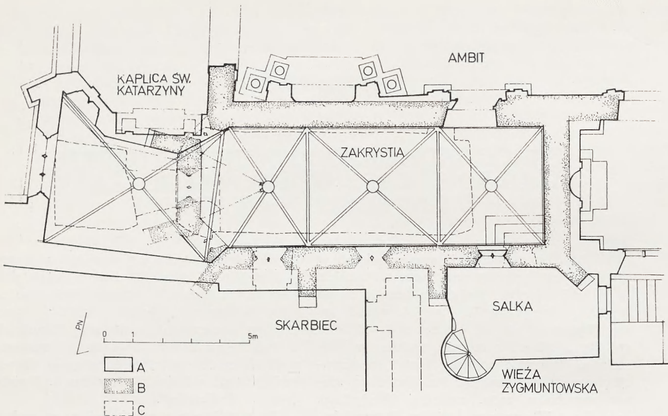
1. Rekonstrukcja rzutu kaplicy Św. Małgorzaty: A. — stan obecny murów przyziemia, B — pierwotny układ kaplicy Św. Małgorzaty, C — krypty, stan obecny. Oprac. P. Stępień
