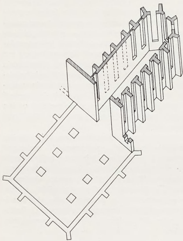
10a. Fazy budowy kościoła Bożego Ciała; kościół w latach 1348—ok.1369 (nadbudowa drewniana została pominięta dla czytelności rysunku)
