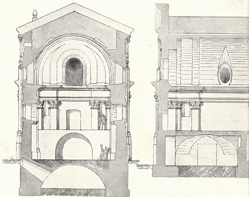
Fig. 2. Kościół św. Agnieszki. —
