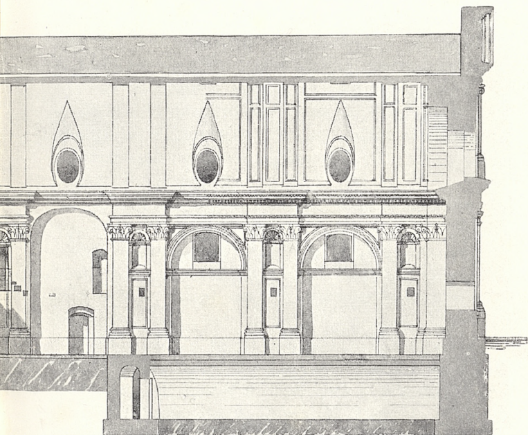
krój poprzeczny i podłużny.
