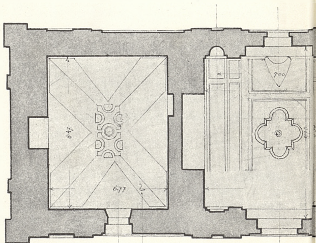
Fig. 1. Kościół św. Agnieszki. — Rzd
