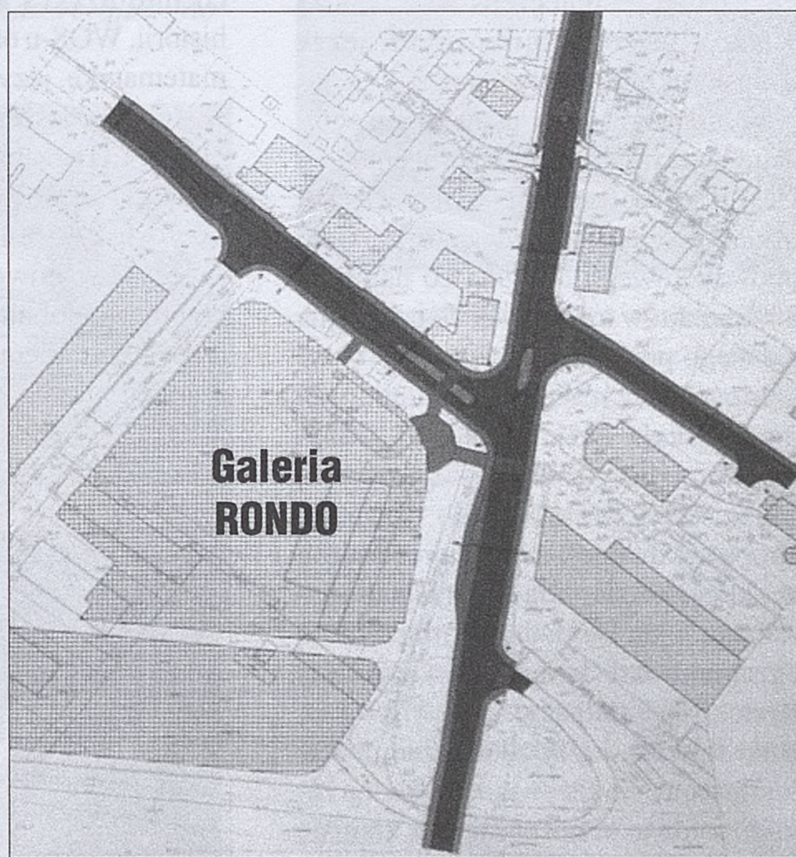
Możliwe rozwiązania komunikacyjne przy powstającej Galerii Handlowej „Rondo” u zbiegu ulic Partyzantów i Proszowskiej. Z lewej projekt rondo, po prawej skrzyżowanie z sygnalizacją świetlną.
