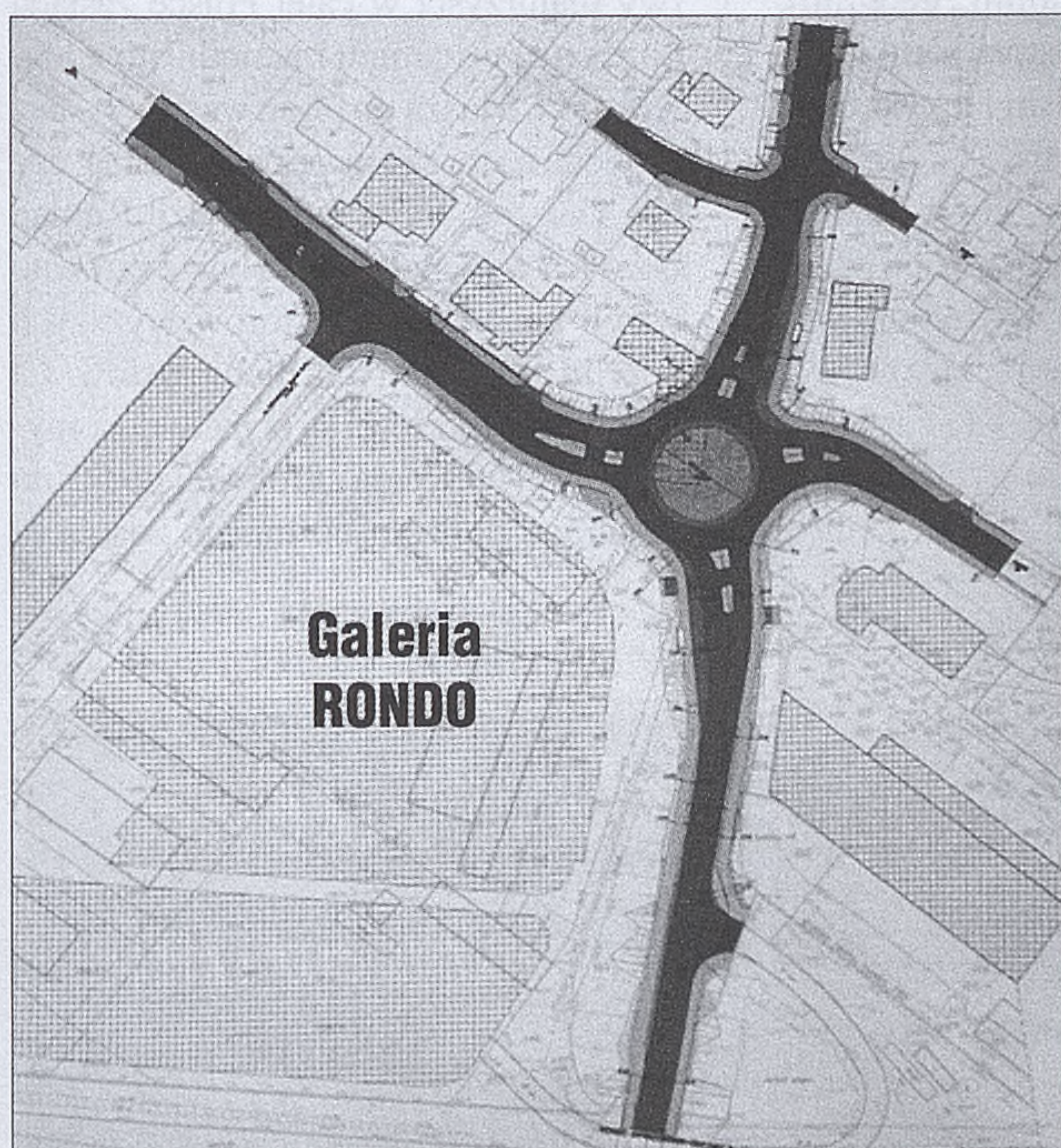
Możliwe rozwiązania komunikacyjne przy powstającej Galerii Handlowej „Rondo” u zbiegu ulic Partyzantów i Proszowskiej. Z lewej projekt rondo, po prawej skrzyżowanie z sygnalizacją świetlną.
