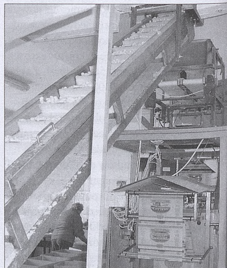
Linia produkcyjna w firmie Jura.
