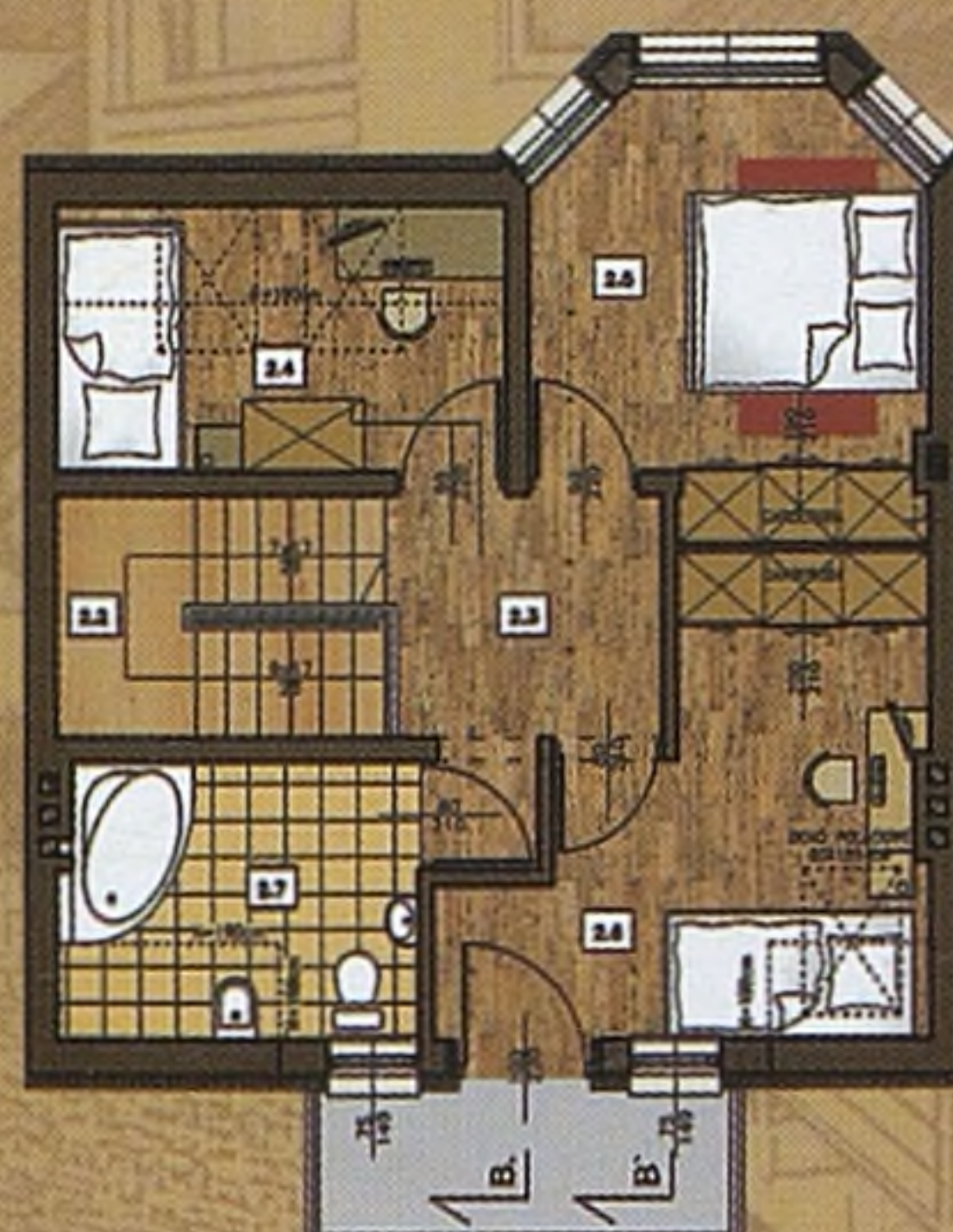
RZUT PODDASZA
