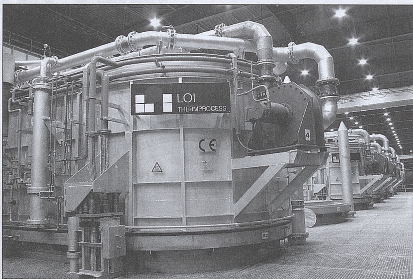
Piece firmy LOI służące do wyżarzania wysokotemperaturowych blach transformatorowych. Zostały oddane do eksploatacji w III kwartale 2006 roku. Dzięki nim firma zwiększyła zdolności produkcyjne blach z 40 do 58 tys. ton/rok.
