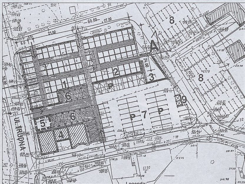
Plan zagospodarowania pl. Gazaris. 1, 2 – hala targowa, 3 – pomieszczenia socjalno-biurowe, 4 – istniejący budynek mieszkalny, 5 – budynek usługowy (przebudowa), 6 – stanowiska do sprzedaży sezonowej, zadaszone lekką konstrukcją, 7 – parking na 50 samochodów, 8 – parking na 54 samochody, 9 – pojemniki na śmieci.
