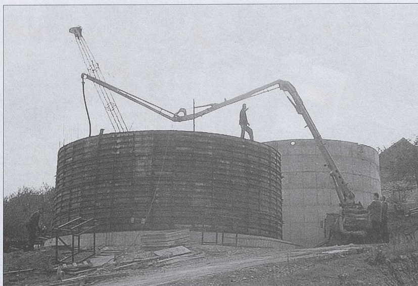
Osiedle Krzęczków II. Budowa dwóch zbiorników do wyrównywania ciśnienia wody dla mieszkańców tego osiedla oraz osiedla Łychów.
