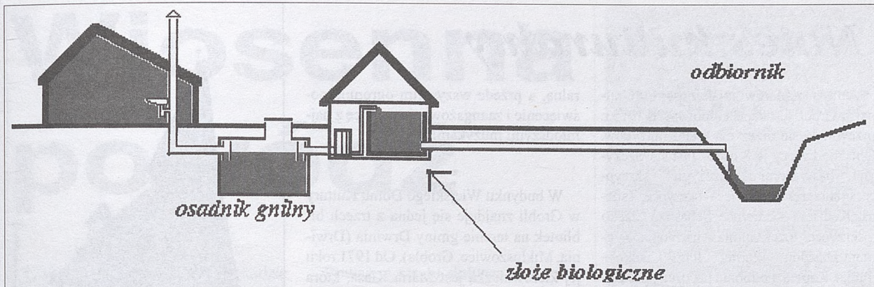
Oczyszczalnia przydomowa ze złożem biologicznym
