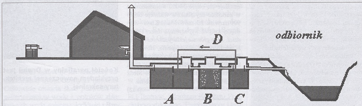
Oczyszczalnia przydomowa z komorą napowietrzania. A, C - osadniki, B - komora osadu czynnego, D - recyrkulacja osadu
