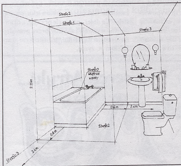
Rys. Podział łazienki na strefy ochronne, w których należy stosować specjalne zabezpieczenia przed porażeniem prądem
