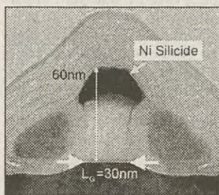
Nowy tranzystor złożony jest z kilku warstw atomów! Fot. Internet
