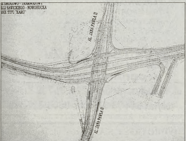
Projekt węzła komunikacyjnego
