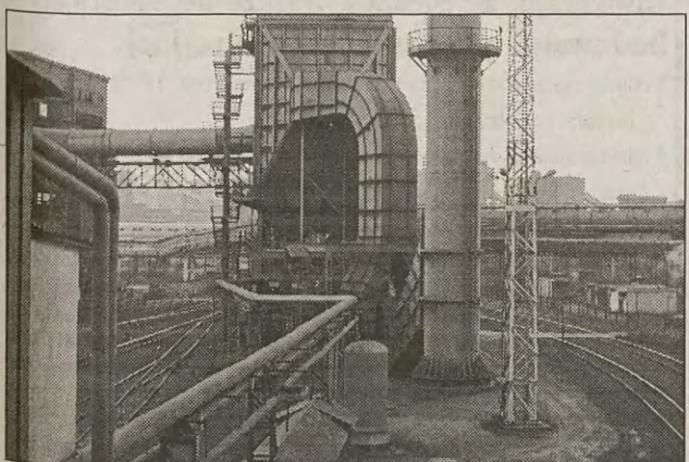
Elektrofiltr hali namiarowej
