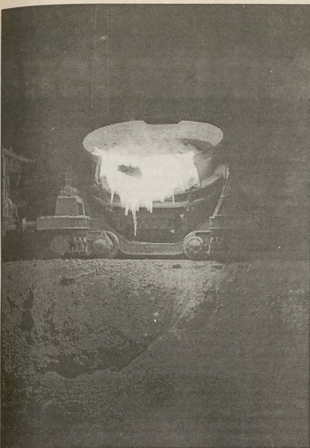
Gorący żużel z wielkich pieców w Hucie im. Sendzimira przewożony jest specjalnymi wagonami na hałdę w Pleszowie, gdzie wylewa się go w głąb wyrobiska
