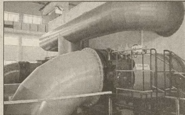
Zakład Uzdatniania Wody RABA w Dobczycach — rurociągi technologiczne
