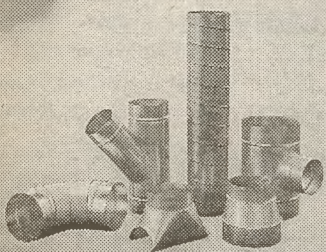
Kanały i kształtki kołowe
