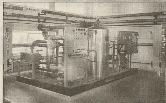
ZUW w Dobczycach — fragment Stacji Ozonowania
