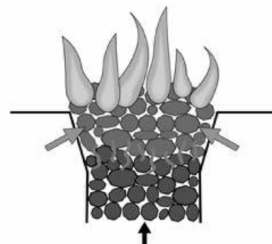
Rys. Kocioł zasypowy spalający przeciwprądowo vs palnik retortowy spalający współprądowo
