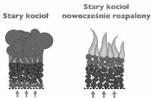
Rys. Kocioł zasypowy spalający przeciwprądowo vs kocioł zasypowy spalający współprądowo
