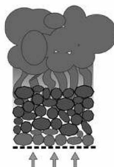
Rys. Kocioł zasypowy spalający przeciwprądowo vs palnik retortowy spalający współprądowo
