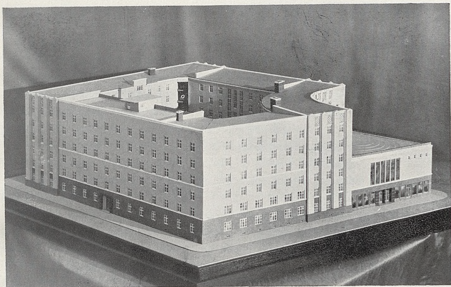
Model domu (widok od strony zachodniej i północnej wraz z narożem t. j. na partję będącą w budowie).
