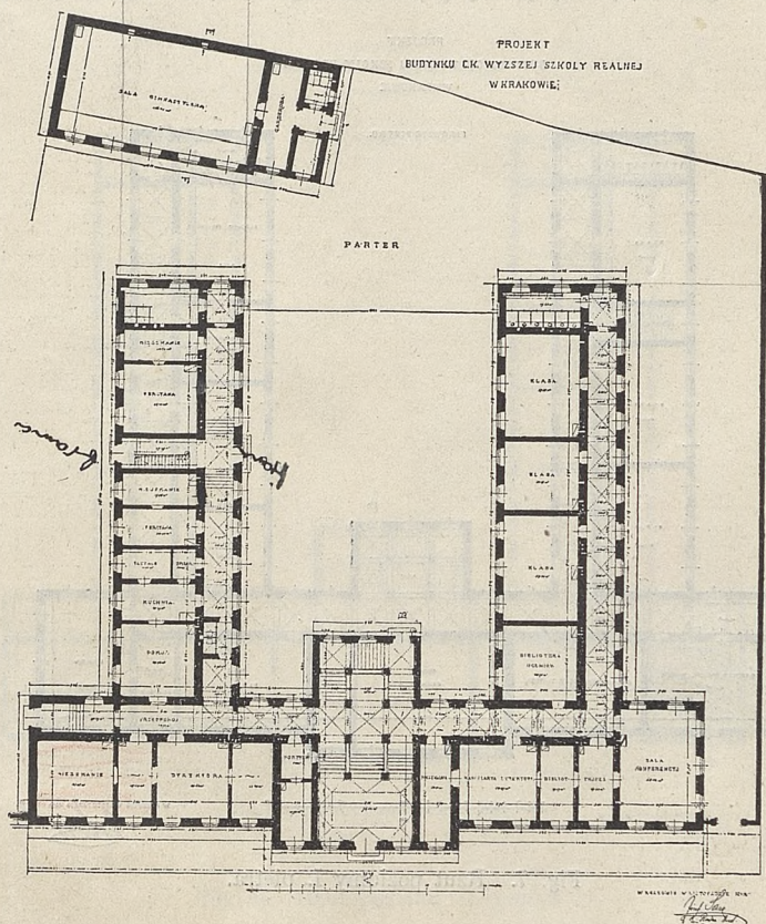
Fig. 6. Rzut poziomy parteru.
