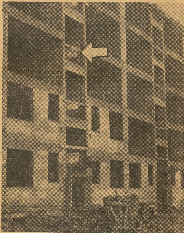
Tu nie będzie ani pieców ani kaloryferów. Blok mieszkalny w Czyżynach, w którym zastosowano płyty grzewcze pomysłu prof. T. Chłipalskiego. (Strzał- ka wskazuje na umiejscowienie jednej z płyt).
