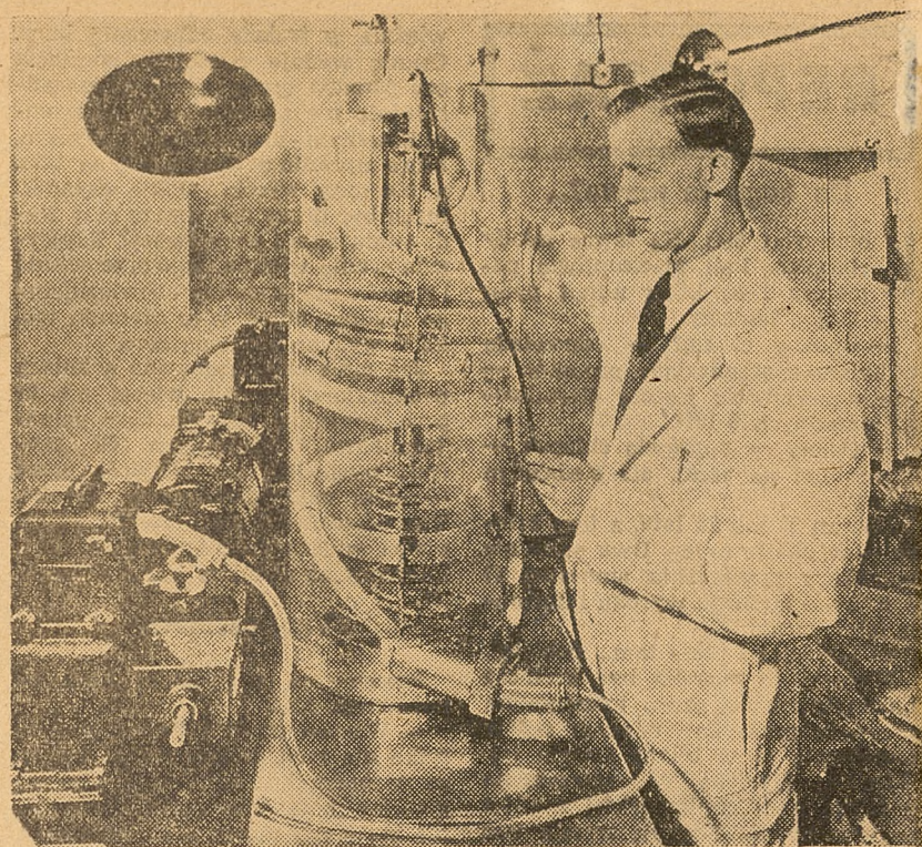
Zbudowano ostatnio w Anglii aparat, zastępujący ludzkie płuca i serce, podczas skomplikowanych operacji chirurgicznych. Konstrukcja aparatu jest podobno niezwykle prosta. Koszt wykonania (przy produkcji seryjnej) nie powinien przekraczać 500 dolarów. Anglicy podają, że metoda zastosowana w konstrukcji aparatu została uprzednio wypróbowana i zastosowana przez naukę radziecką.
