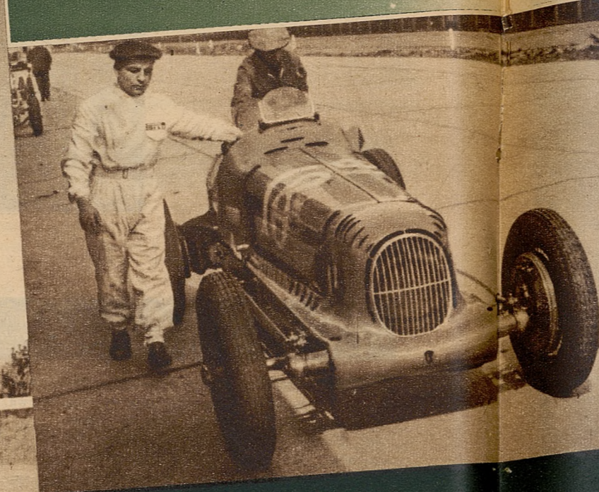
Poniżej od lewej ku prawej: 1) Nadzieja Francji: sportowy lekki wóz 1.5 l. Talbot, poddawany jest obecnie nowym próbom. 2) Sensacyjne rozwiązanie podwozia Auto-Union: silnik kompresorowy w tyle, rama z rur o wadze... 36 kg. 3) Stara, ale b. szybka angielska maszyna ERA będzie w tym roku gruntownie przebudowana.
