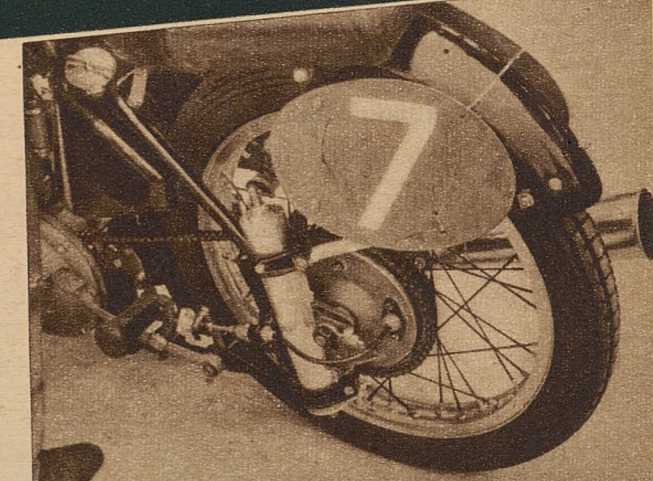
Dla podniesienia zalet drogowych stosują Angliki w swych motocyklach resorowanie tyłu. Na zdjęciu konstrukcja fabryczna Excelsior 250 ccm
