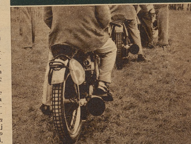
Dla podniesienia wydajności swych silników stosował Norton lekki wydechowy przy wylotach rur, niewidzianych dotychczas wielkich wymiarów
