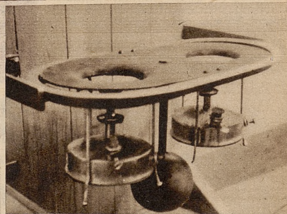
Dwie kuchenki, umieszczone w ten sposób, że utrzymują się zawsze w pionie, mimo wahań jachtu.
