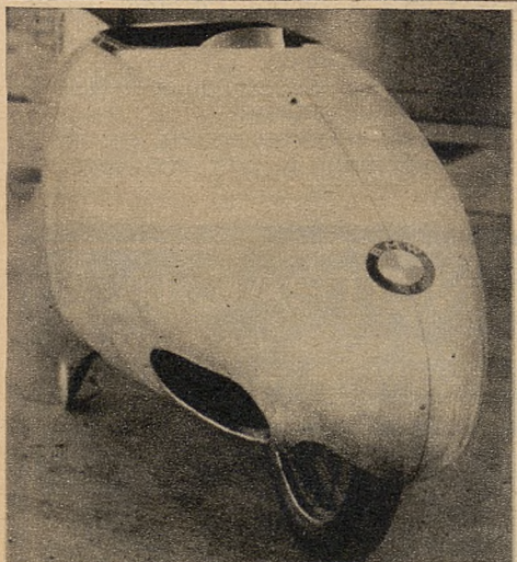
Najnowszy typ „półpancernego“, aerodynamicznego motocykla, widziany od przodu, na którym Henne ustanowił rekord świata 279.5 km na godzinę.
