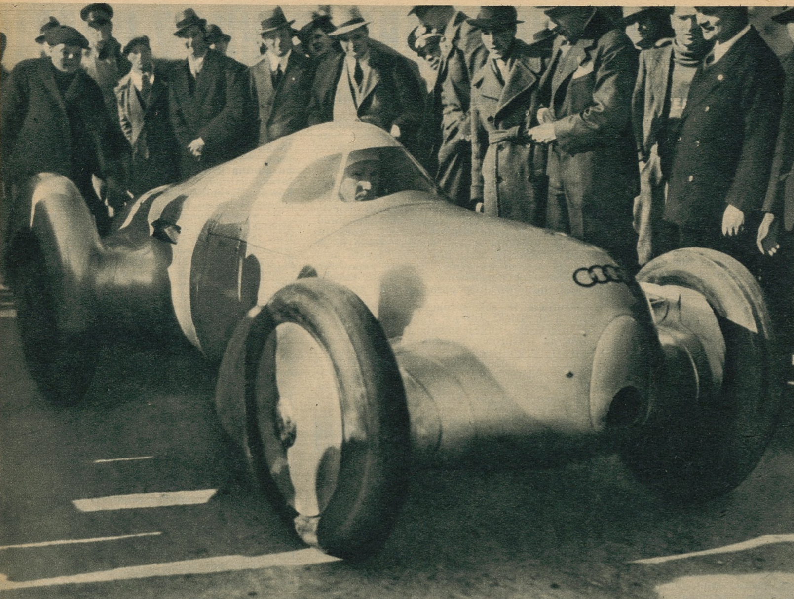
Nowy typ wozu wyścigowego Auto-Union 16-to cylindrowy, z silnikiem z tyłu. Karoserja zamknięta jest nowością przy wozach wyścigowych.
