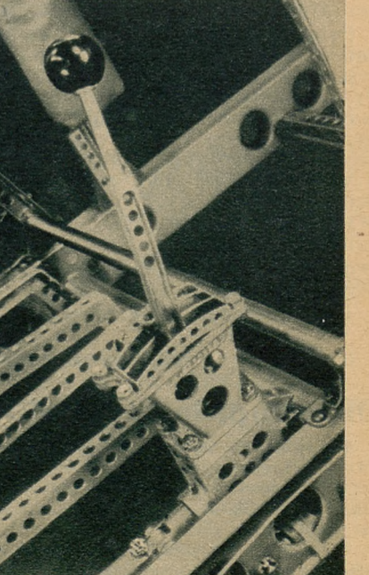
Nowa konstrukcja wozów niemieckich, w której stosuje się ramy dziurkowane, celem zmniejszenia ciężaru.
