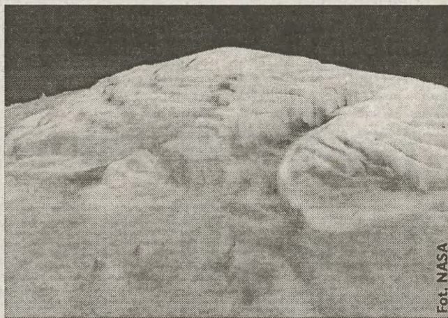
Tak wygląda lodowa czapa polarna bieguna północnego na Marsie. Jej obraz został zrekonstruowany na podstawie ostatnich pomiarów ukształtowania terenu planety przez sondę kosmiczną „Mars Global Surveyor”
