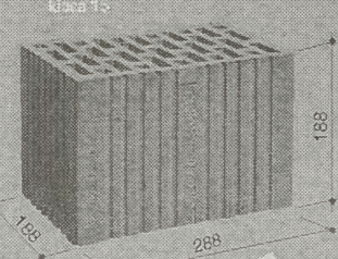
PUSTAK SZ 188
