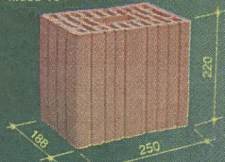
PUSTAK U 220 klasa 15
