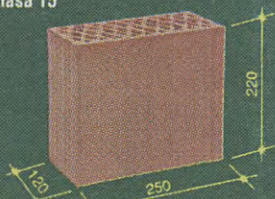
CEGLA KRATÓWKA K-3 klasa 15
