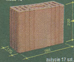
CEGLA MODULARNA klasa 15
