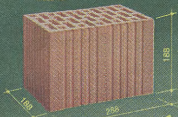
PUSTAK S2 188 klasa 15
