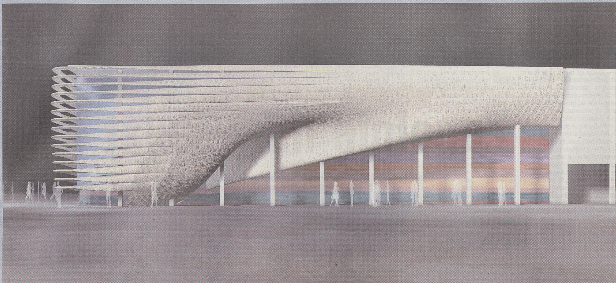
Fasada pawilonu polskiego. – Za pomocą nowoczesnego oprogramowania komputerowego modelowana jest forma fasady. Na podstawie tych rysunków przygotowane zostaną formy stalowe, które następnie oplecione zostaną białą wikliną. Zajmą się tym rękodzielnicy – wyjaśnia Krzysztof Ingarden.
