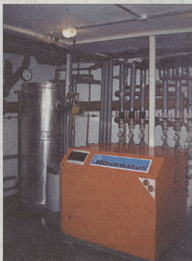
Pompa ciepła Hibernatus-Wadowice w budynku wielorodzinnym na osiedlu Bemowo w Warszawie
