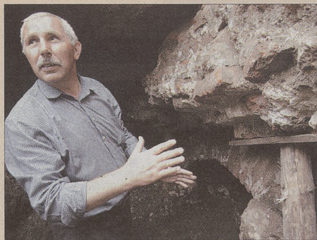
Emil Zaitz przy podstemplowanym fundamencie kolumnady Sukiennic
