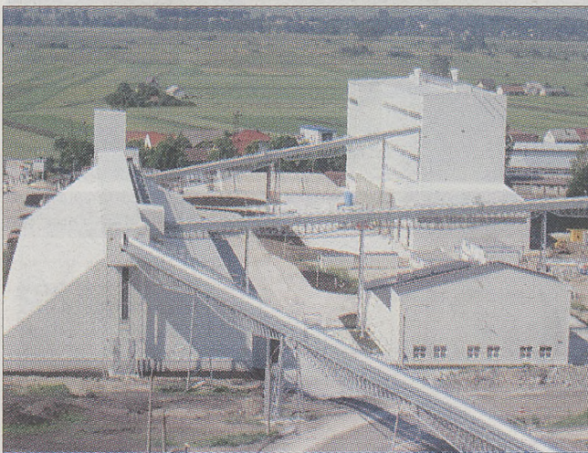
Koszt 54 mln zł uruchomiono nową prażalnię gipsu w Leszczach, która zapewnia otrzymywanie najwyższej jakości półproduktów gipsowych
