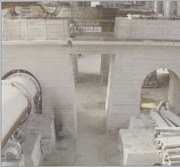
Bonarka – żelbetowa hala pieców
