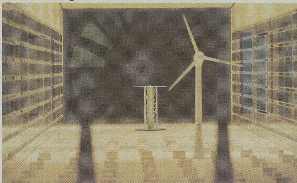
Tunel aerodynamiczny w Laboratorium Inżynierii Wiatrowej PK
